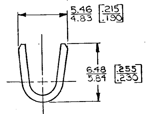
SECT A-A
